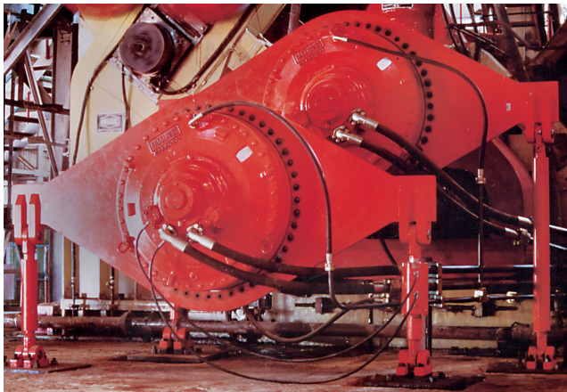
Högtryckscylinder för tung hydrauldraft High pressure cylinders for heavy applications
